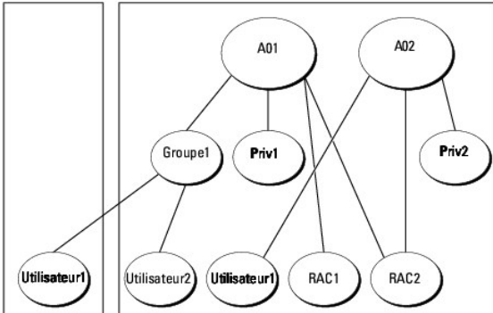
Figure 6-5. Accumulation de privilèges pour un utilisateur
