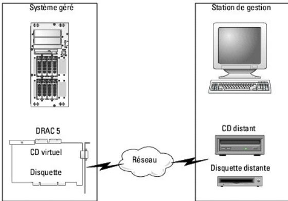
Figure 11-1. Architecture globale d'un média virtuel
